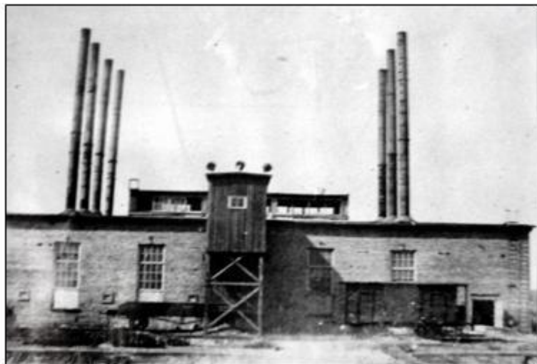
Первоначальное энергетическое хозяйство завода № 77 состояло из двух паровозов. Фото 1943 г. из фондов музея школы № 49.
