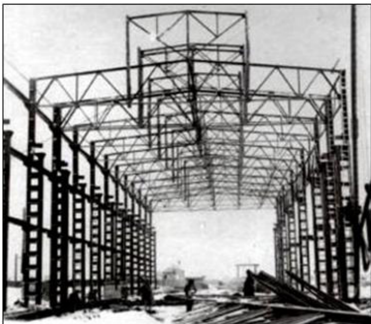
Строительство Барнаульского котельного завода. Каркас главного первого цеха. Фото 1943 г.
